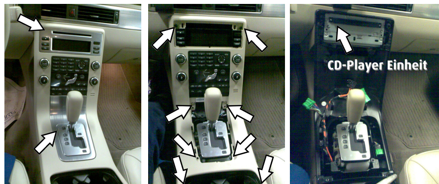
Abb.: Ausbau der Mittelkonsole im Volvo V70
